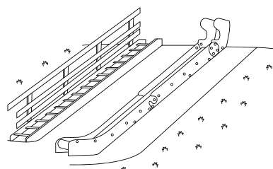
Glissoire simple droite sur talus
